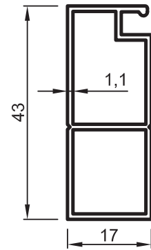
No : 3916 Büyük Sineklik 0,415 kg/m
