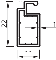
No : 2554 Küçük Sineklik 0,190 kg/m
