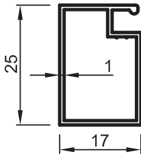
No : 3263 Büyük Sineklik 0,210 kg/m
