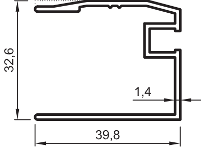
No : 5199 (*) Sineklik Profili 0,490 kg/m
