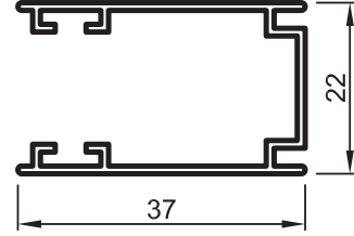
No : 5702 Sineklik Profili 0,330 kg/m
