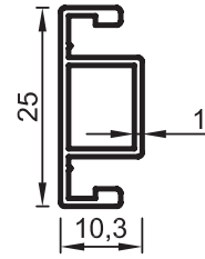
No : 6581 Sineklik Profili 0,215 kg/m
