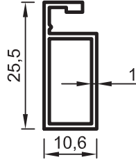
No : 5159 Küçük Sineklik 0,210 kg/m
