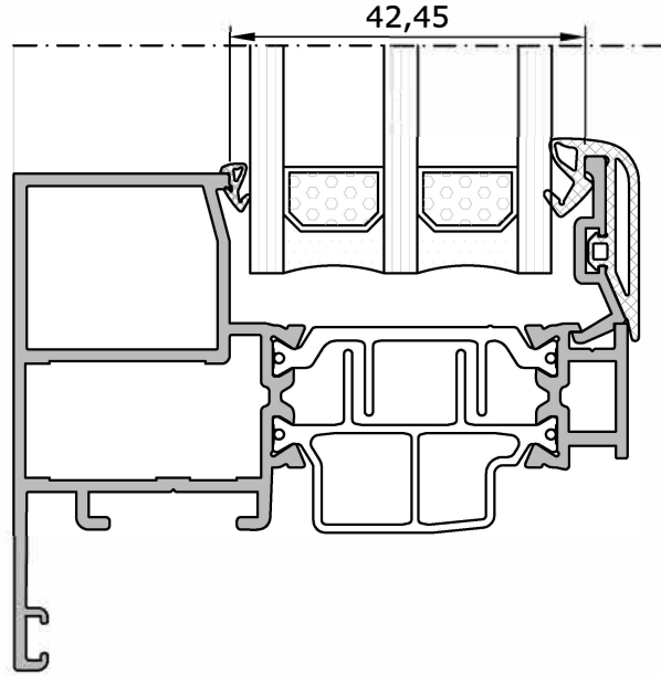
GİZLİ KANAT İÇİN CAM ÇITASI VE FİTİL TABLOSU / GLAZING BEAD AND GASKETS TABLE FOR HIDDEN VENT
